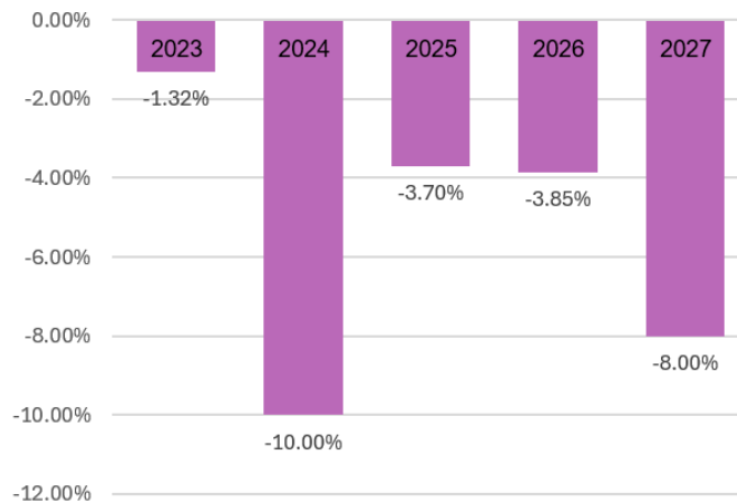
BI Tools
